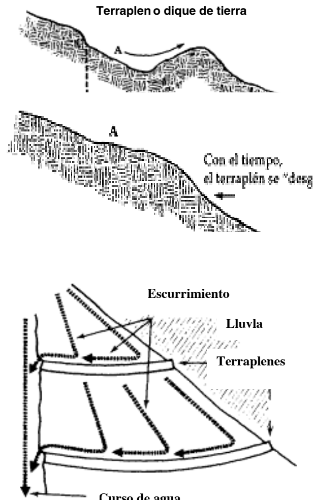
Figura 6. Construcción de un sistema de conservación del suelo
