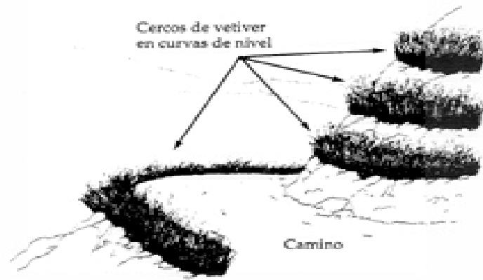
Figura 41. Protección de los bordes de los caminos
